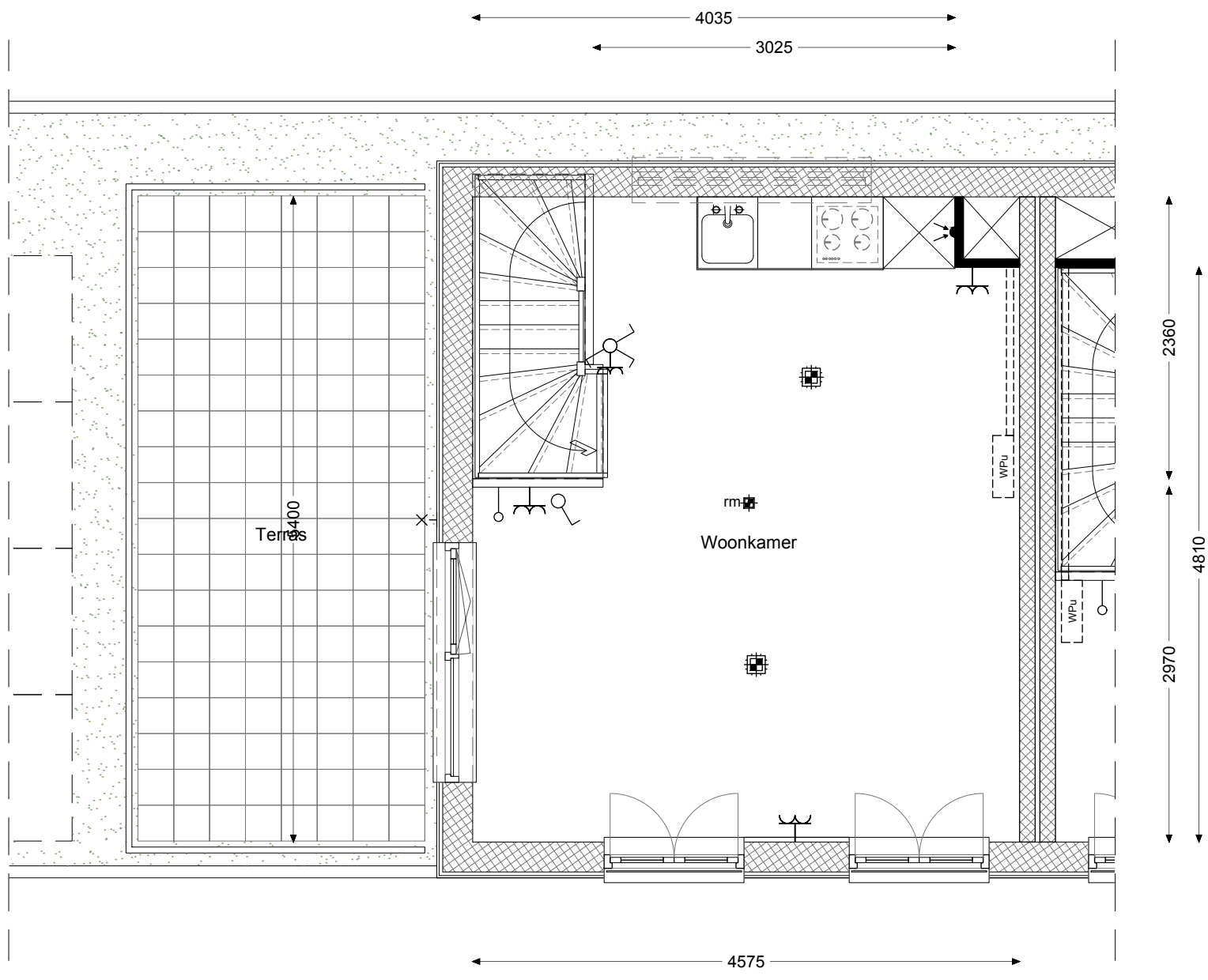
Eerste etage
