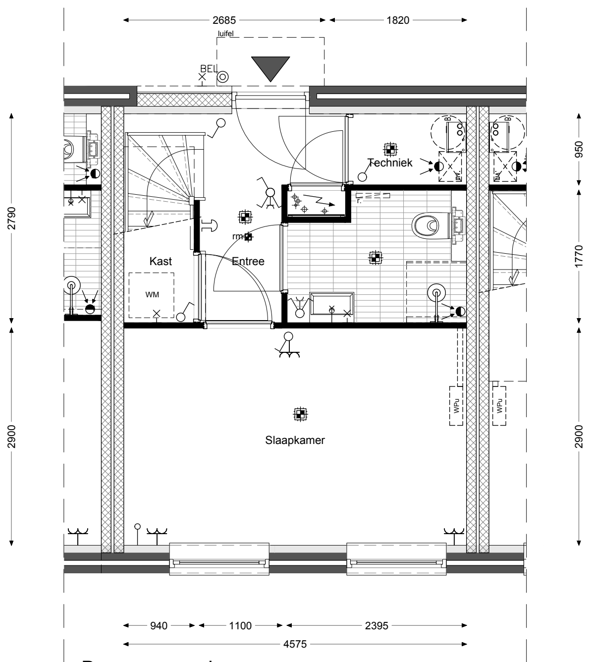
Begane grond
