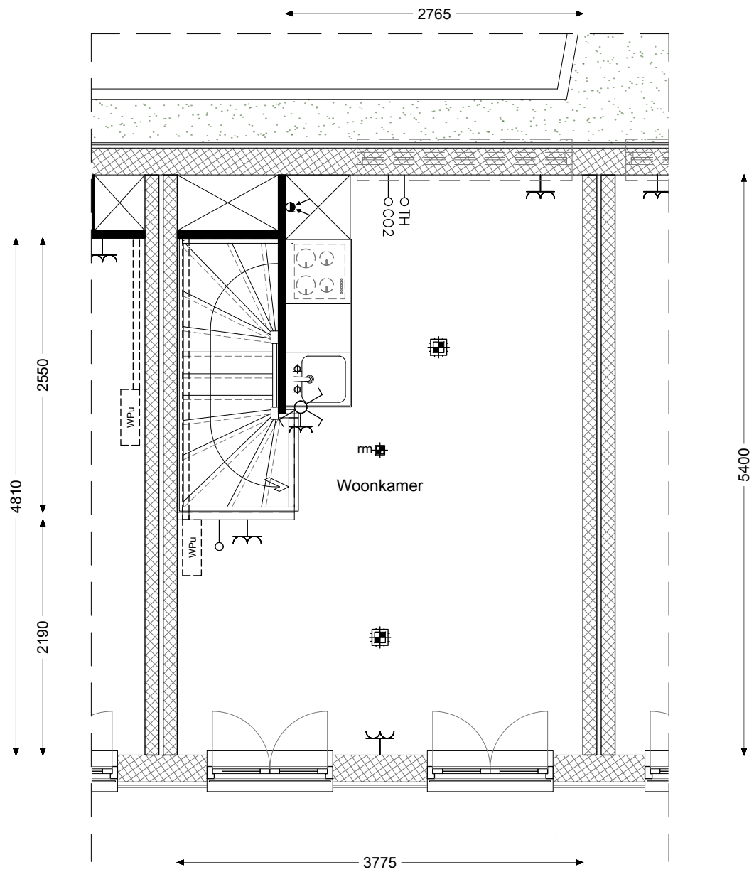
Eerste etage
