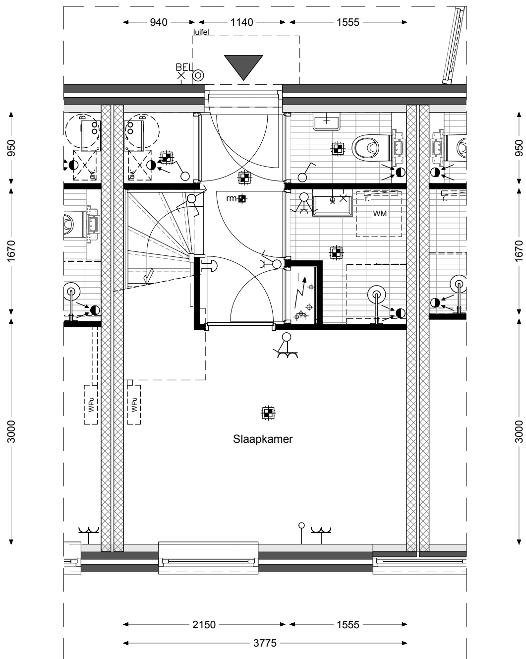
Begane grond
