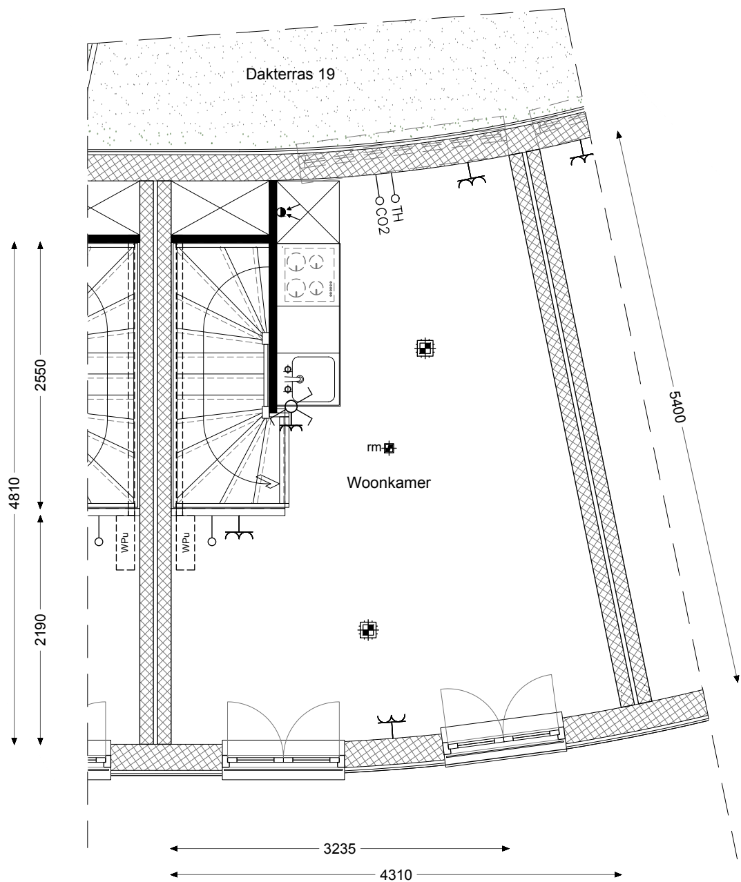
Eerste etage
